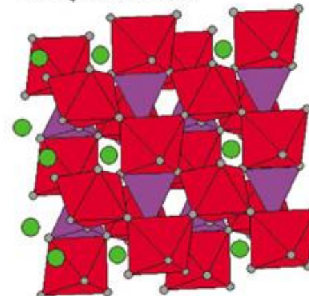
\text{LiFePO}_4 : olivine structure
