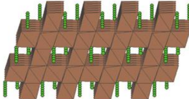
\text{LiMn}_2\text{O}_4 : spinel structure
